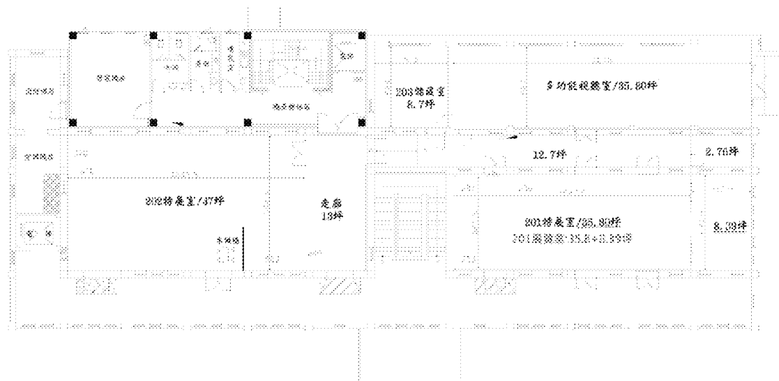
貳層平面圖
